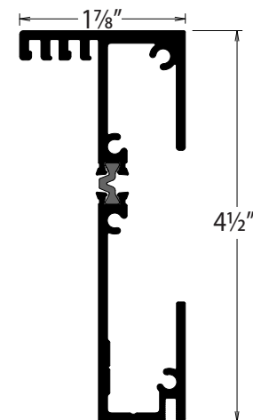
JAMB E0021
