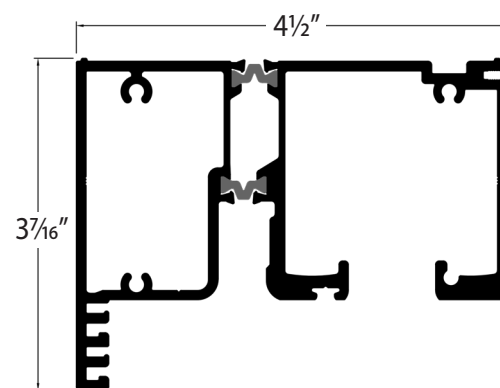
HEADER E0020
