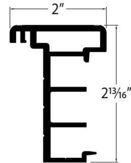
ASTRAGAL E0029
