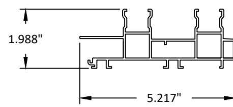
37 OPTIONAL 5/8" RISER ADD ON 6063-T5
