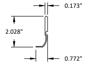
35 OPTIONAL 1" RISER ADD ON 6063-T5
