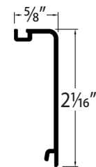
END CAP
