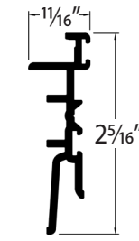
P HOOK
