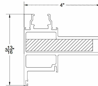
ASTRAGAL
