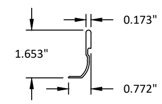
37 OPTIONAL 5/8" RISER ADD ON 6063-T5
