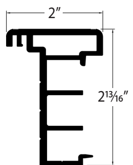
ASTRAGAL E0029
