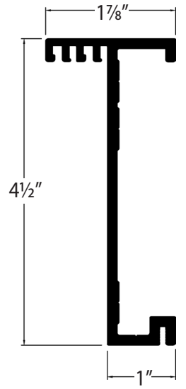
JAMB E0033
