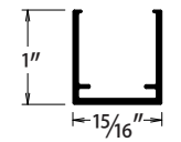
ADA SILL | E0128
