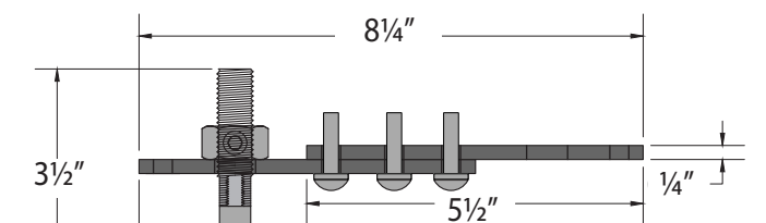
BOTTOM PIVOT PIN
