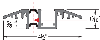
ADA Sill
